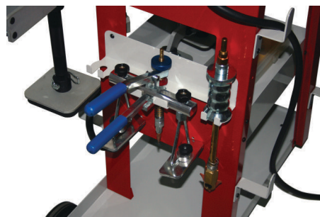
Rückansicht der Ausbeulstation CEBOPULL Junior
